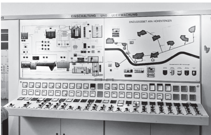
Aufnahme Betriebswarte
