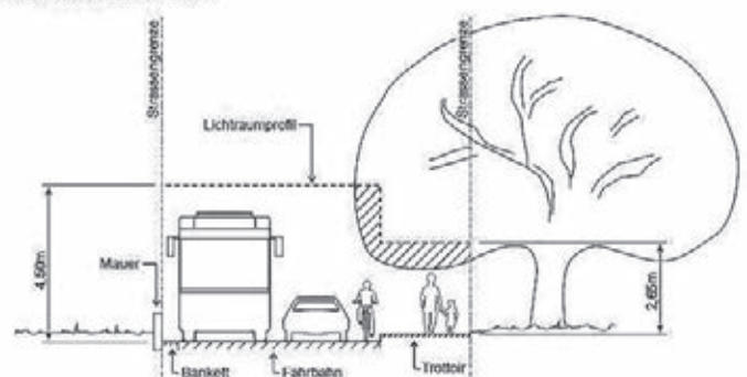
A: Lichtraum in der Höhe
