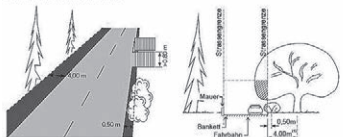
B: Minimale seitliche Abstände
