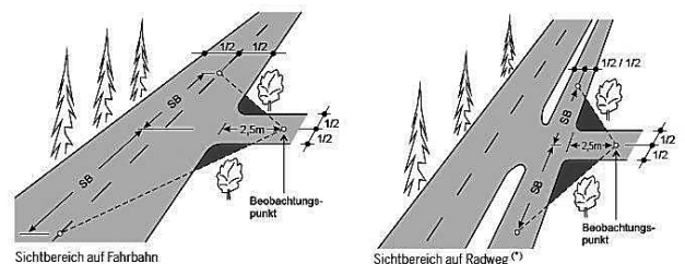
C: Minimal freizuhaltende Sichtbereiche Knotenbereich (Einmündungen und Kreuzungen)
